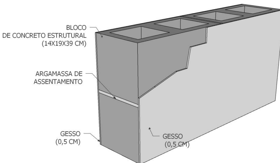
Figura 1 - Esquema do elemento construtivo, objeto dessa FAD
