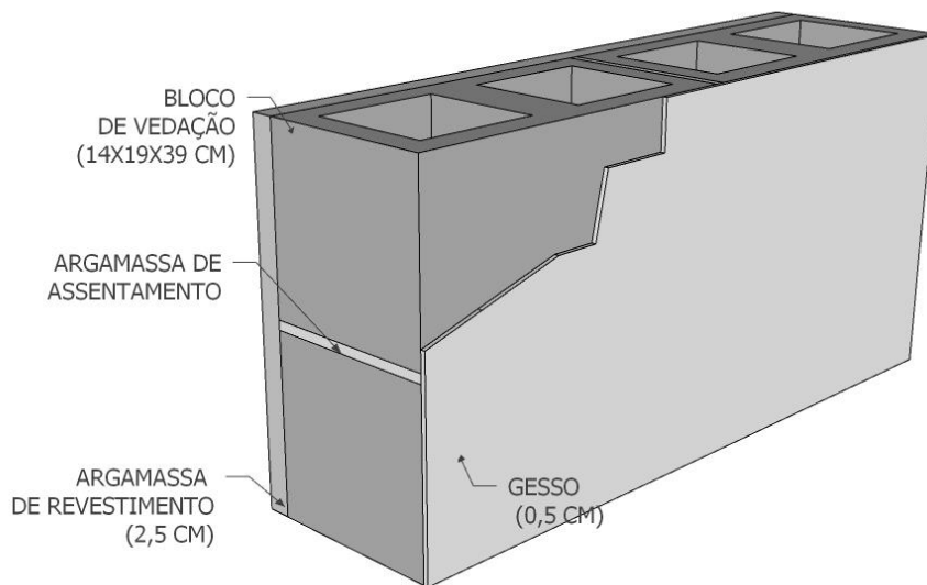
Figura 1 - Esquema do elemento construtivo, objeto dessa FAD
