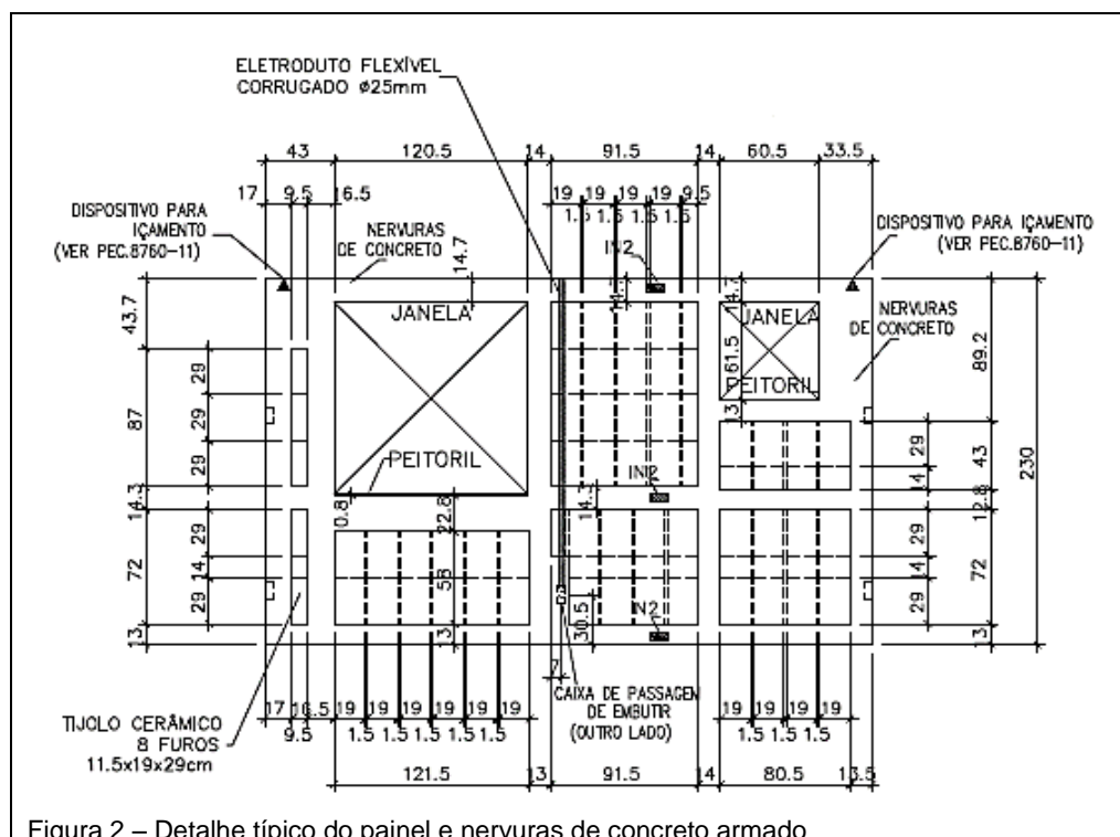
Figura 2 – Detalhe típico do painel e nervuras de concreto armado
