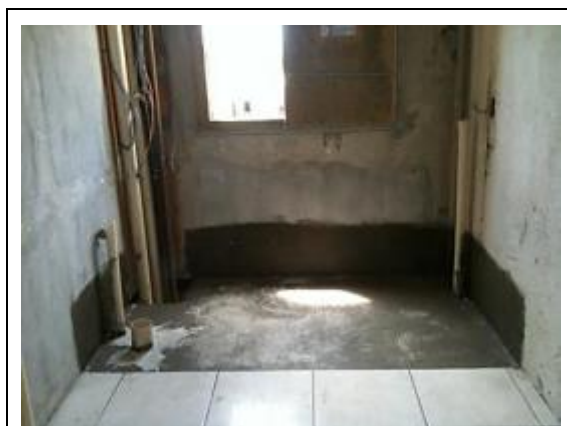
Figura 35 – Impermeabilização laje de concreto e barrado de 300mm na parede
