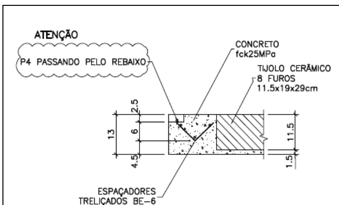
Figura 29 – Detalhe das ligações (medidas em cm)
