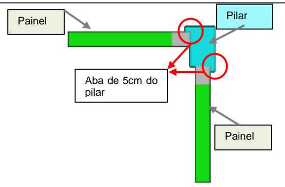
Figura 28 – Detalhe da interface painel-pilar
