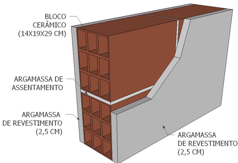
Figura 1 - Esquema do elemento construtivo, objeto dessa FAD
