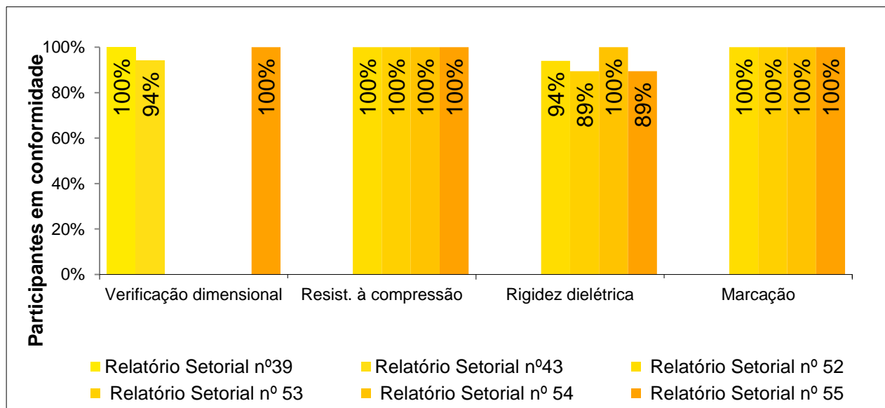
Figura 2 – Evolução do percentual de aprovação das fábricas de empresas participantes (eletrodutos flexíveis “leve”)
