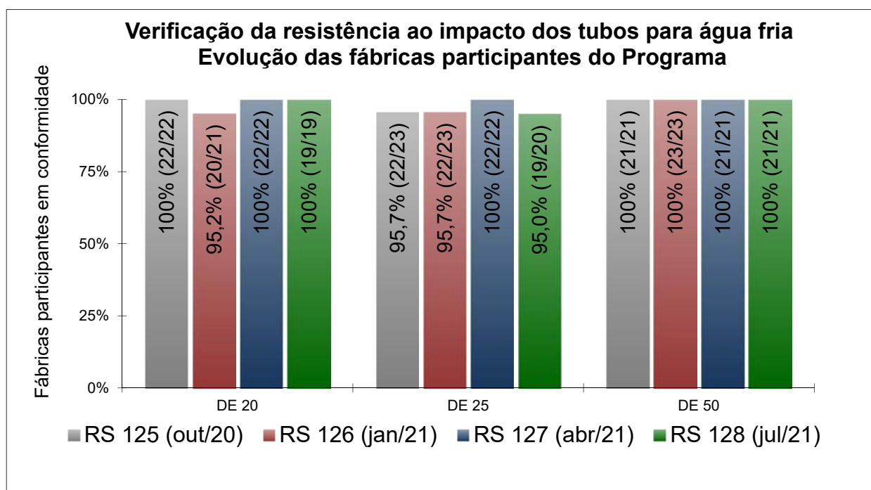
Figura 6 - Verificação da resistência ao impacto a 0°C dos tubos para água fria DE 20, DE 25 e DE 50
