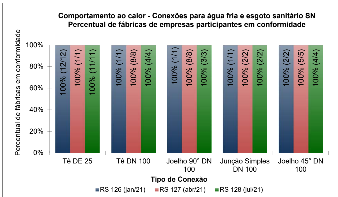
Figura 10 - Verificação do comportamento ao calor das conexões para água fria e esgoto sanitário SN
