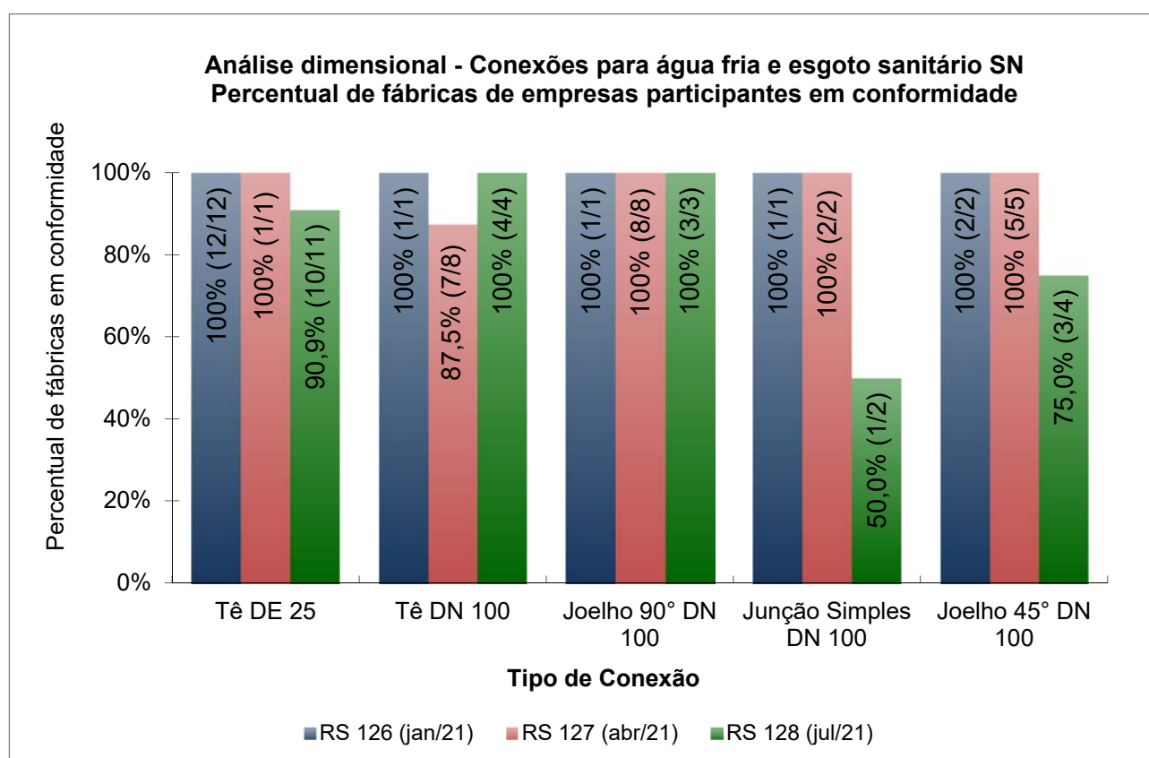
Figura 9 - Análise dimensional de conexões para água fria e esgoto sanitário SN
