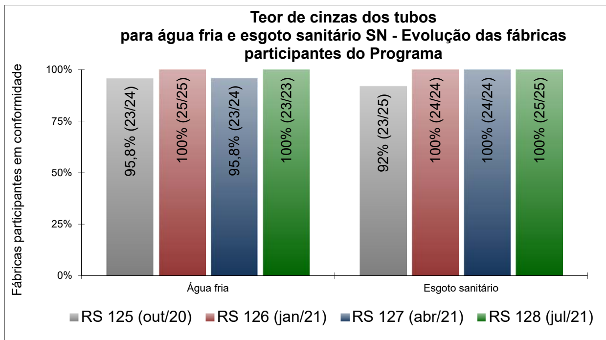
Figura 3 - Teor de cinzas do composto dos tubos para água fria e esgoto sanitário SN
