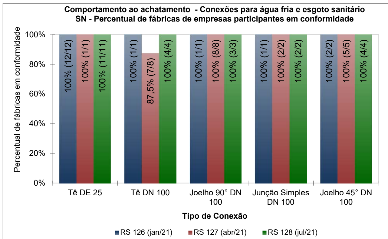
Figura 11 - Verificação do comportamento ao achatamento das conexões para água fria e esgoto sanitário SN
