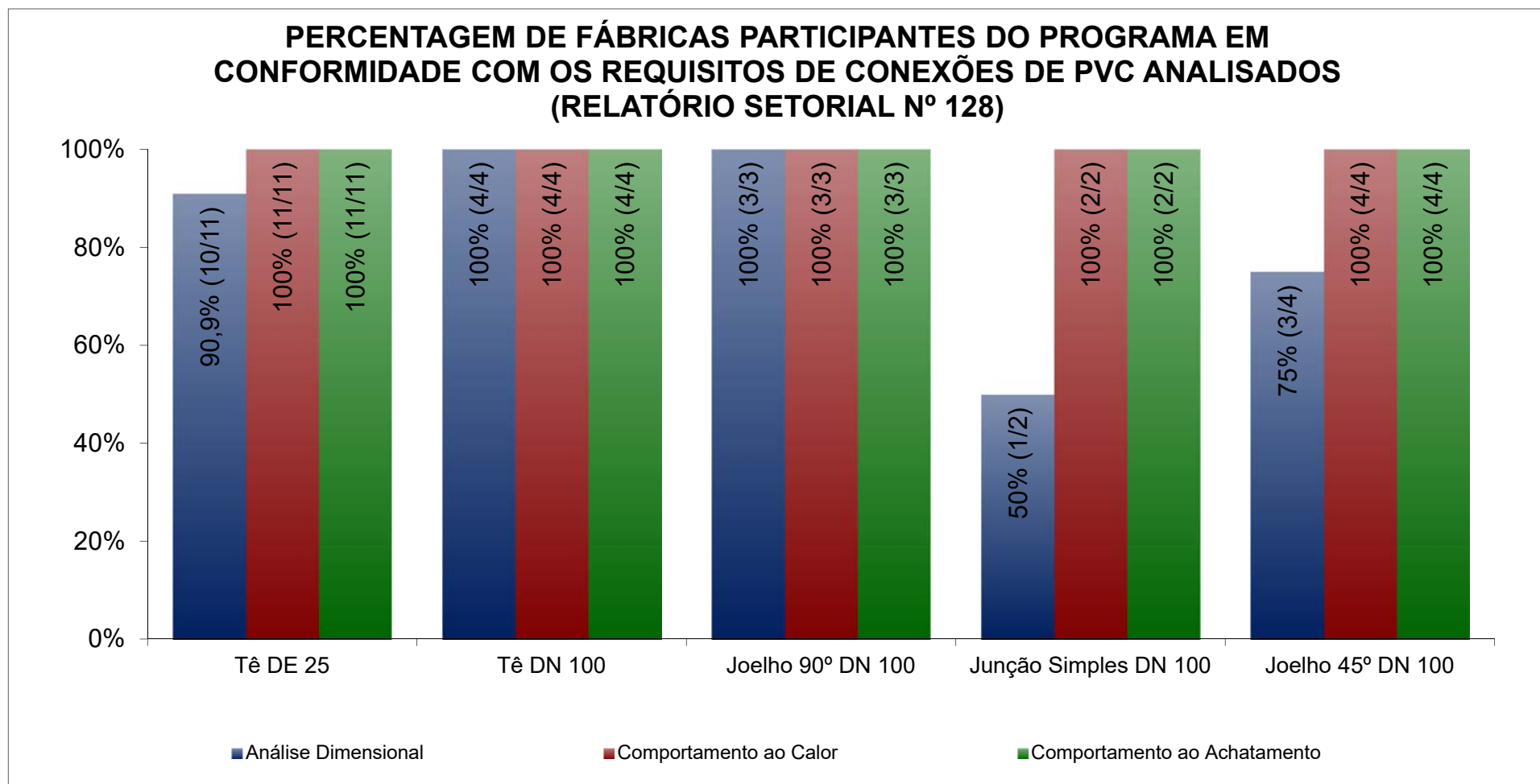
Figura 12 - Conexões de PVC - Fábricas participantes em conformidade com os requisitos analisados pelo Programa Setorial da Qualidade – Relatório Setorial nº 128
