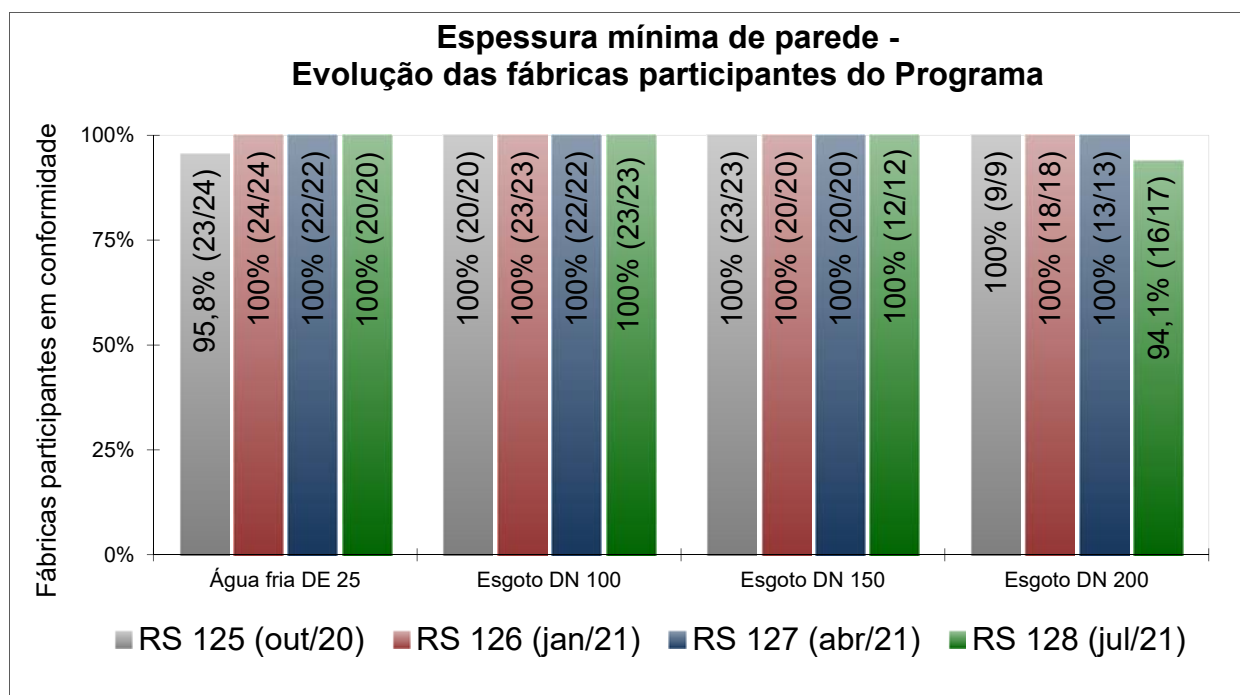
Figura 2 - Espessura de parede dos tubos para água fria DE 25 e tubos para esgoto sanitário DN 100, DN 150 e DN 200
