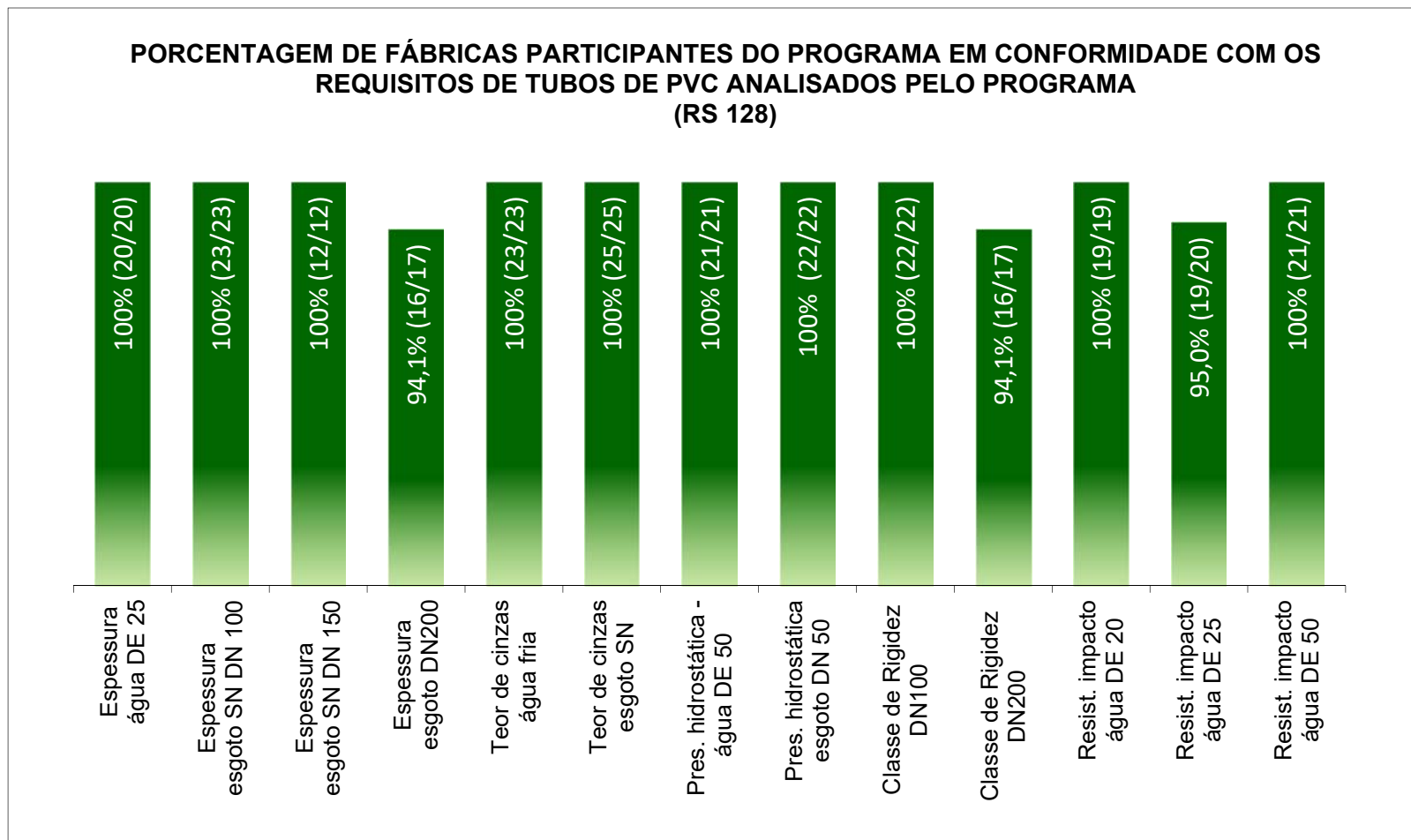
Figura 8 - Tubos de PVC - Fábricas participantes em conformidade com os requisitos analisados pelo Programa Setorial da Qualidade – Relatório Setorial nº 128
